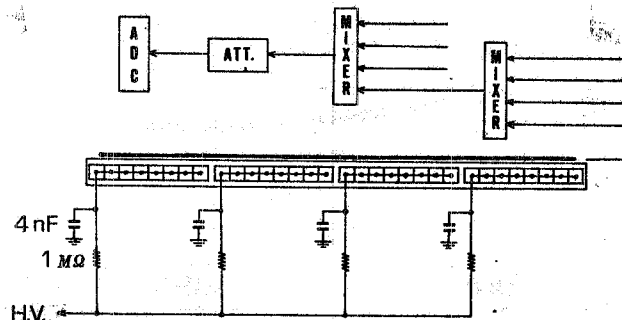
FIG. 4 - H.V. and readout scheme.
