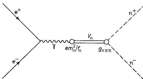
Fig. 1. - Diagram for e^+e^- \rightarrow V_n \rightarrow \pi^+\pi^- .
