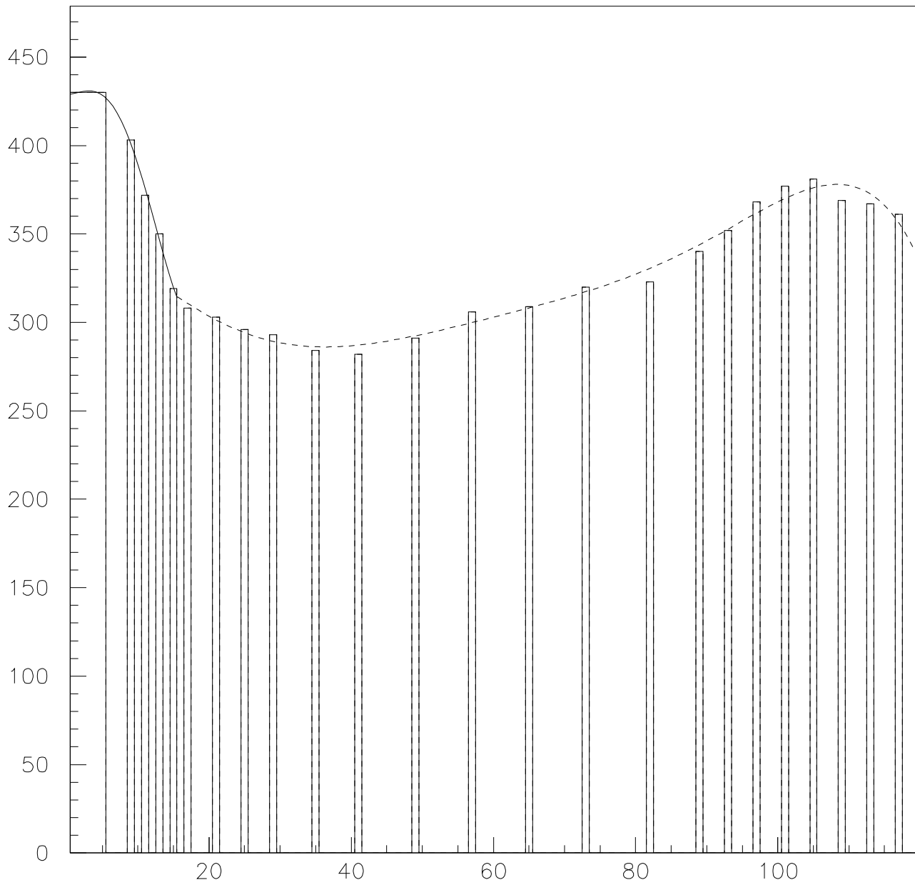
WIRE SAG (micron) VS LAYER
