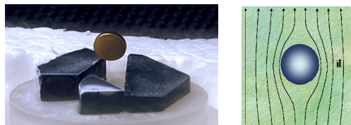
Fig.2 Levitazione magnetica di un magnetino (0.1 Tesla) su alcuni campioni di YBCO alla temperatura dell'azoto liquido (77K). La foto evidenzia l'espulsione del campo magnetico dal materiale superconduttore ceramico ad alta temperatura critica (effetto Meissner). Foto LNF-INFN (laboratorio LAMPS)
