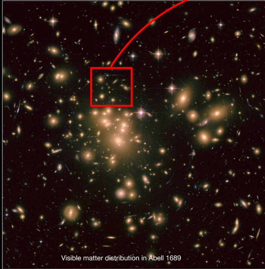
Abell 1689
