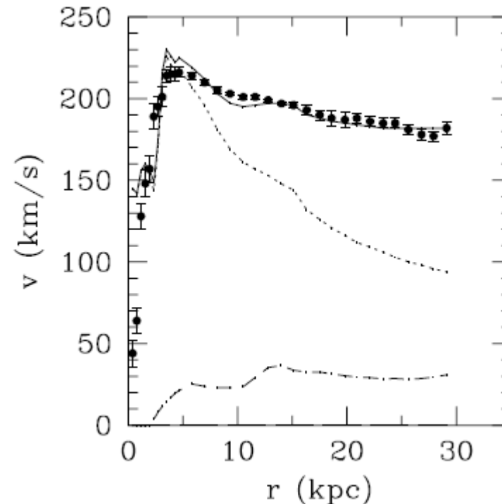
NGC 2903
