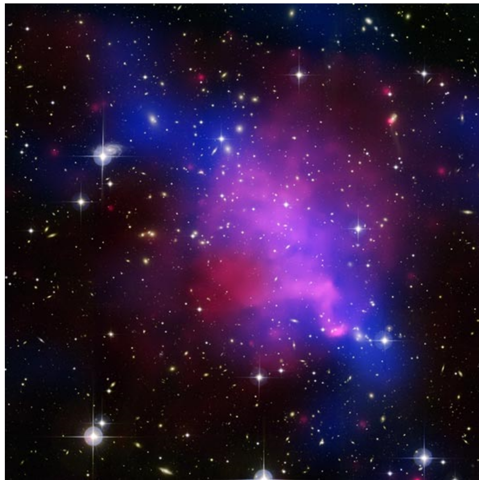
Abell 520
